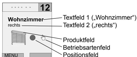
Abb. 2 Display im Betriebsmodus (Beispiel 2): Kanal 12, eingelernte Jalousie, STOPP-Zustand, Handbetrieb aktiv; Textfeld 1 (hier „Wohnzimmer“) und Textfeld 2 (hier „rechts“) individuell eingetragen
