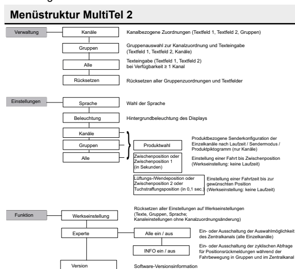
Abb. 4 Menüstruktur des MultiTel 2
